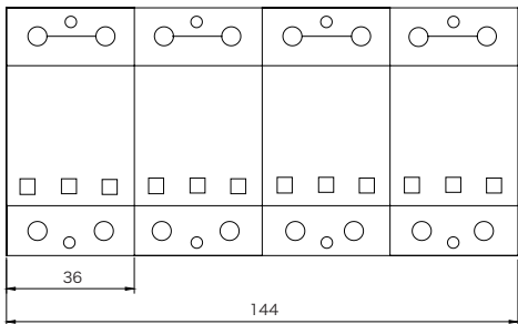
YAP1-80 外形尺寸
