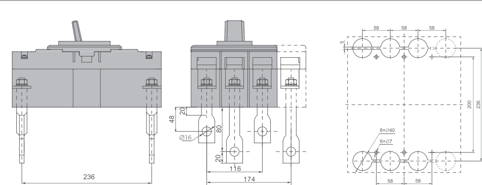
APEM6 – 630 板后接线尺寸（三极、四极）X-X、Y-Y 三极断路器中心 6
