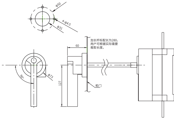
630A 及以下手柄辅助尺寸
