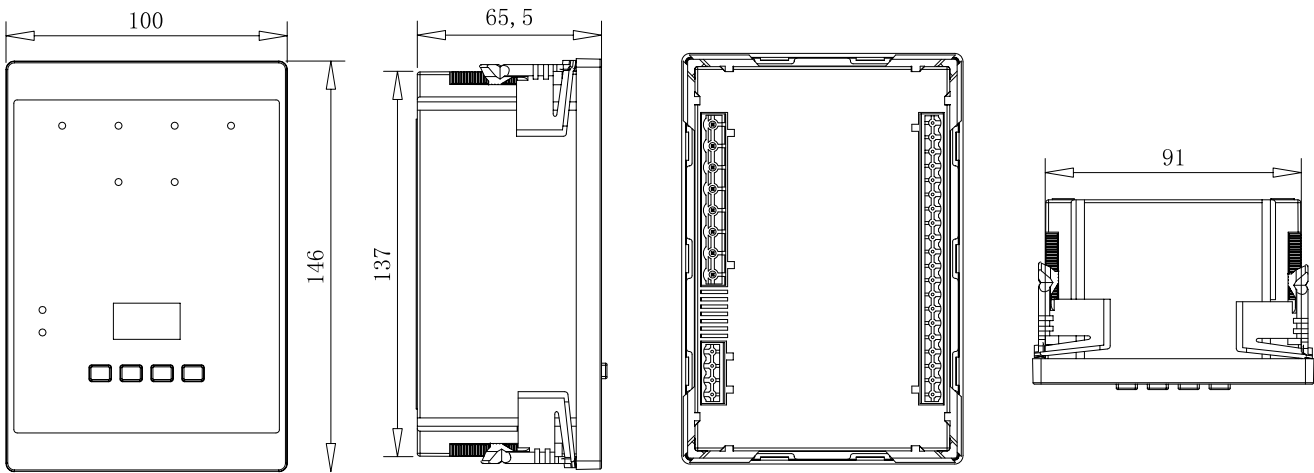
APEK3 型智能控制器开孔尺寸示意图
