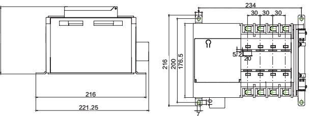
APEQ5-125 外形尺寸
