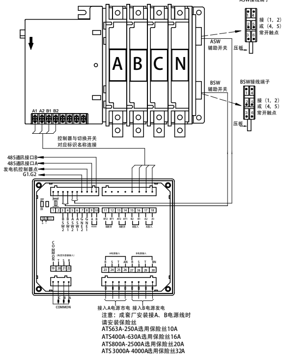
APEK1 配合 APEQ2 双电源接线示意图
