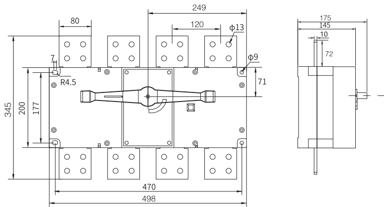
3200A 3 极 外形安装尺寸图
