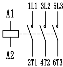
AC1-185~330接线图
