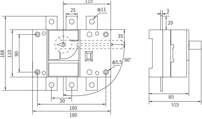
250A 3 极 外形安装尺寸图
