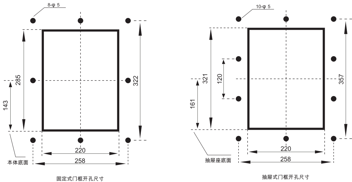
AW11-1600 门框尺寸及开孔尺寸
