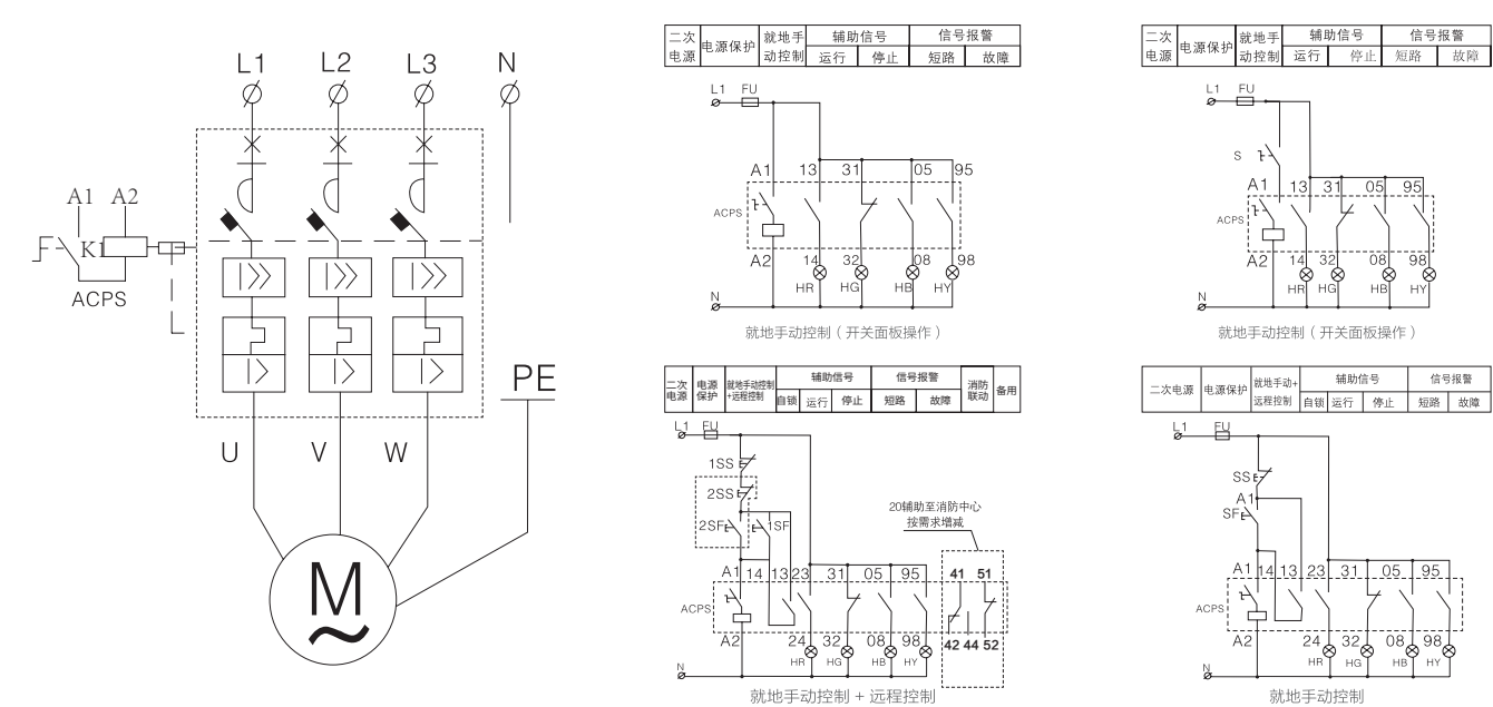
接线示意图
