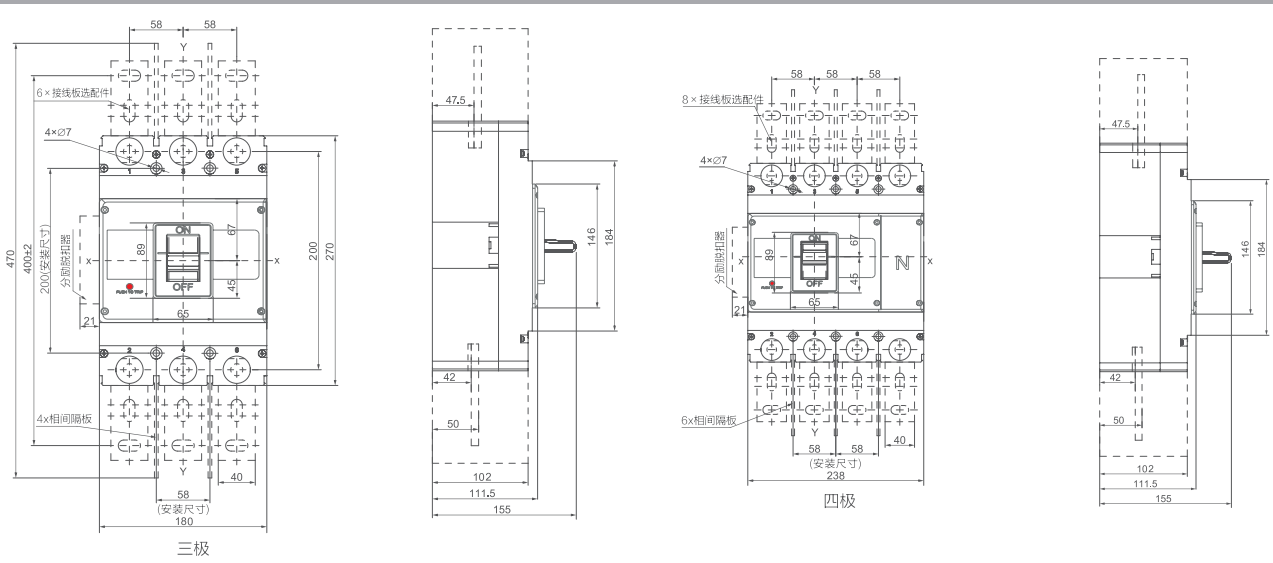
APEM6 – 630 板前接线尺寸（三极、四极）X-X、Y-Y 三极断路器中心
