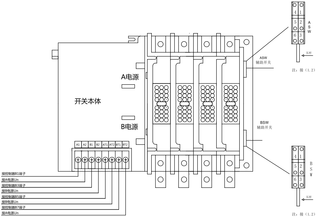
APEQ5 配外置控制器接线图
