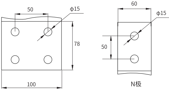
3200A 铜排辅助尺寸
