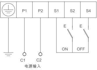
CD2型电动操作机构接线图
