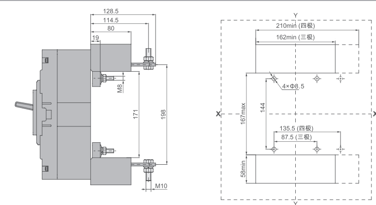
APEM6 – 400 插入式接线尺寸（三极、四极）X-X、Y-Y 三极断路器中心
