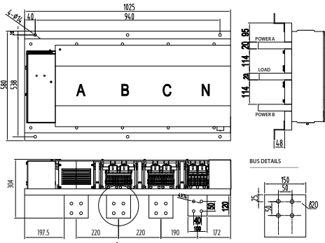
APEQ3-4000A-4
