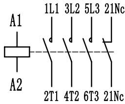
AC1-09~32/01接线图
