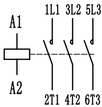
AC1-115~170接线图
