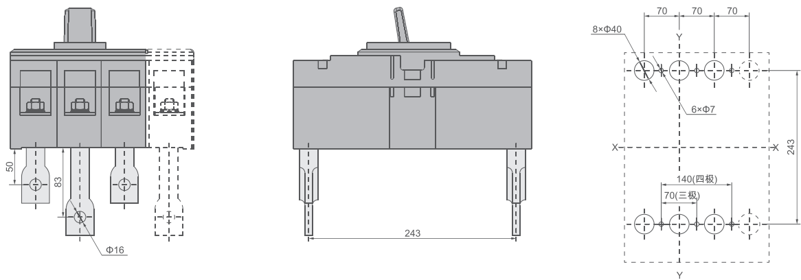
APEM6 – 800 插入式接线尺寸（三极、四极）X-X、Y-Y 三极断路器中心
