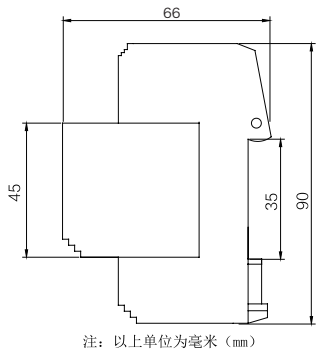
YAP1-65 外形尺寸
