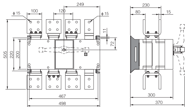
3200A 4 极 外形安装尺寸图
