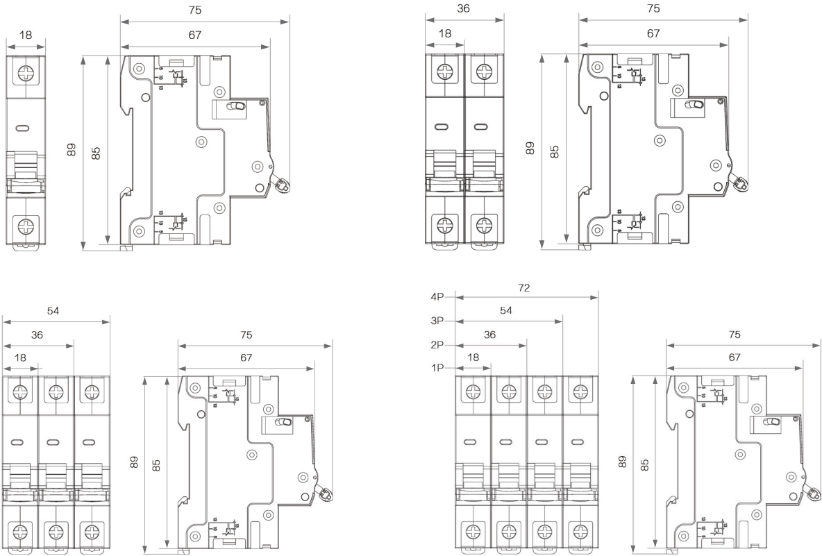
ASCB2 外观尺寸图
