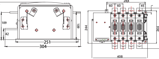
APEQ5-800 外形尺寸
