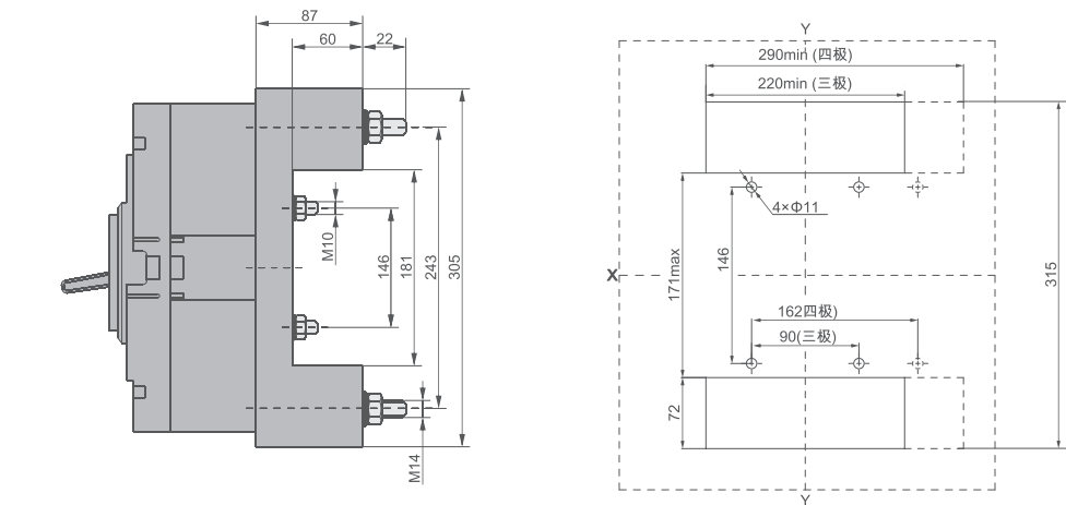
APEM6 – 800 插入式接线尺寸（三极、四极）X-X、Y-Y 三极断路器中心
