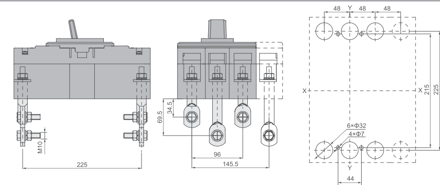
APEM6 – 400 插入式接线尺寸（三极、四极）X-X、Y-Y 三极断路器中心
