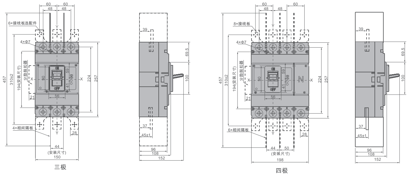
APEL6-400 系列板前接线外形尺寸及安装尺寸
