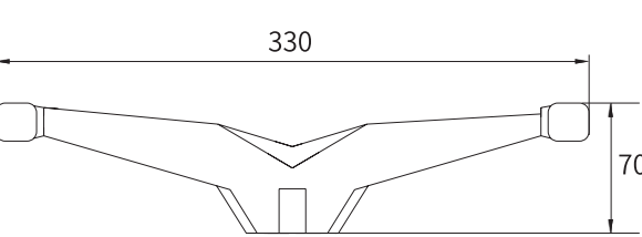
1600A-3200A 手柄辅助尺寸
