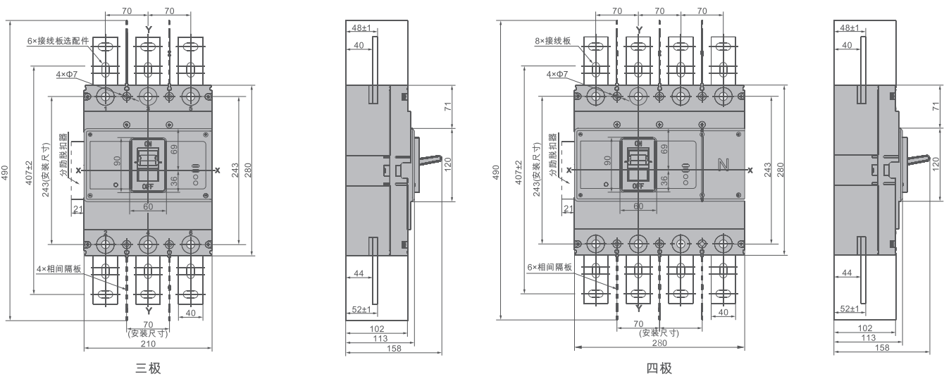
APEL6-630 系列板前接线外形尺寸及安装尺寸
