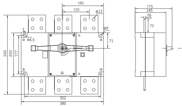
1600A 4 极 外形安装尺寸图
