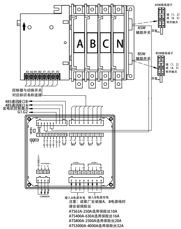
APEK1 配合 APEQ3 (500A 以上) 双电源接线示意图
