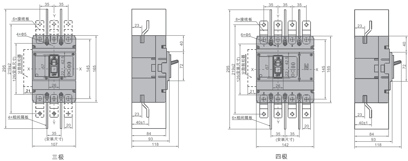
APEL6-250 系列板前接线外形尺寸及安装尺寸
