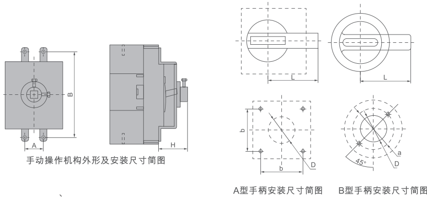
手动操作机构外形及安装尺寸图
