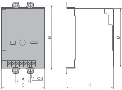
电动操作机构外形尺寸及安装尺寸 表十一
