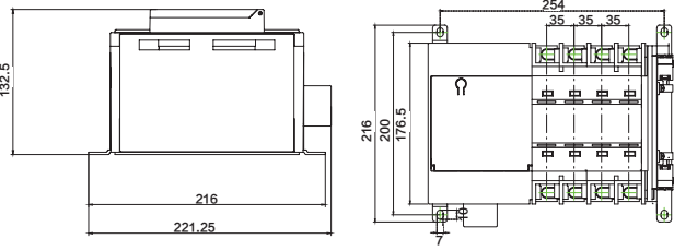
APEQ5-250 外形尺寸
