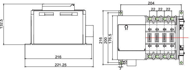
APEQ5-63 外形尺寸
