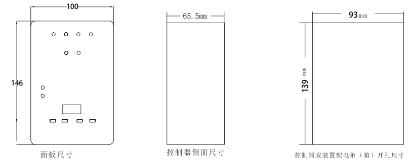
APEK3 标准控制器开孔尺寸示意图
