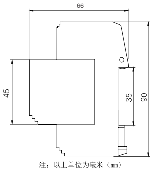
YAP1-40 外形尺寸
