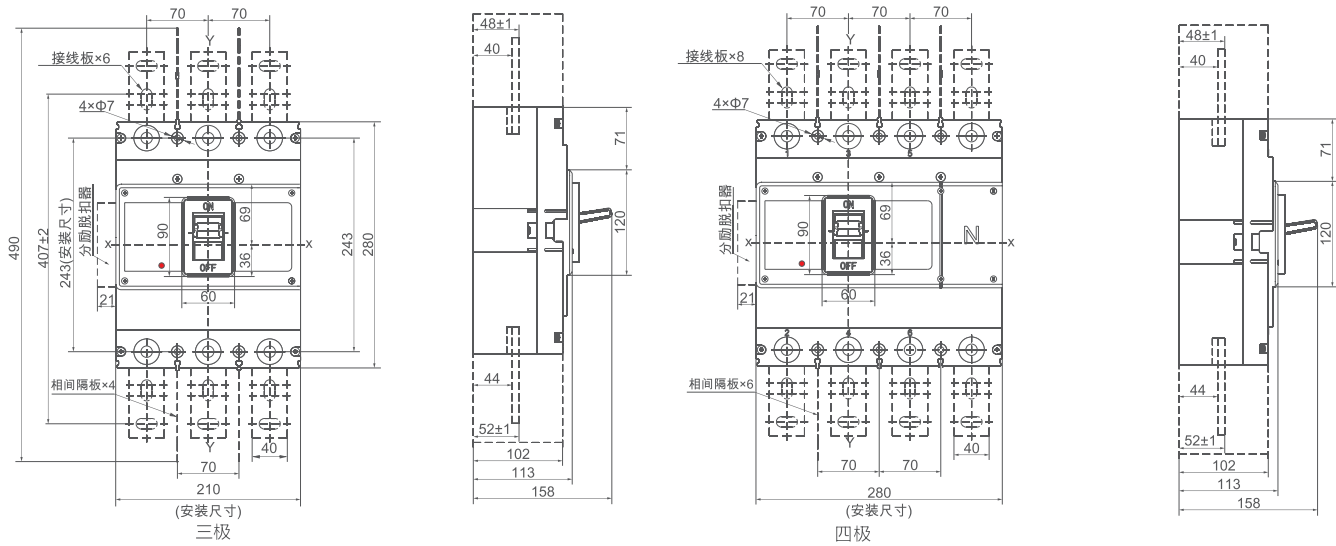
APEM6 – 800 板前接线尺寸（三极、四极）X-X、Y-Y 三极断路器中心
