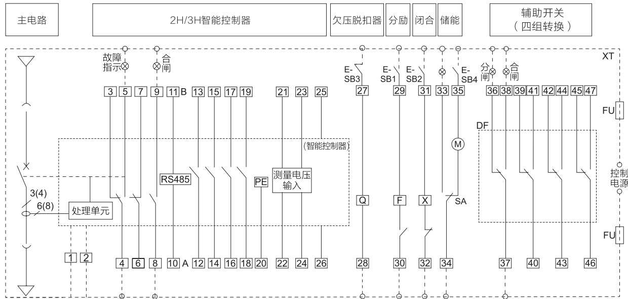
控制回路接线图 (2H\3H )
