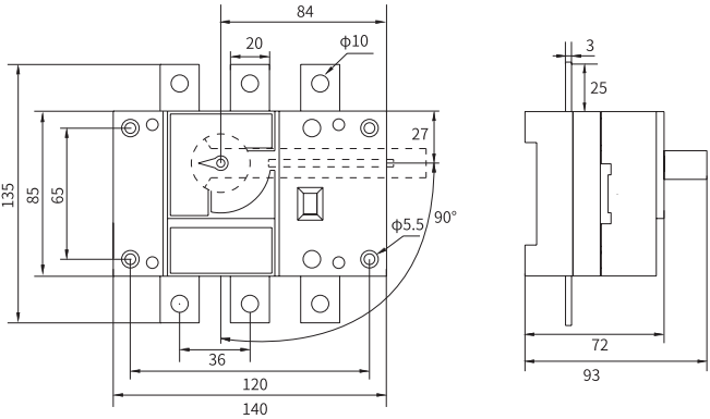
160A 3 极 外形安装尺寸图
