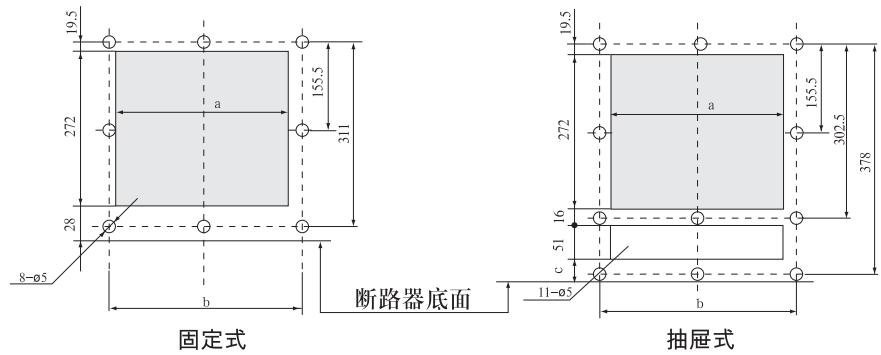
2000 型及以上壳架门框尺寸及开孔尺寸
