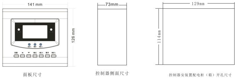
APEK2 标准控制器开孔尺寸示意图
