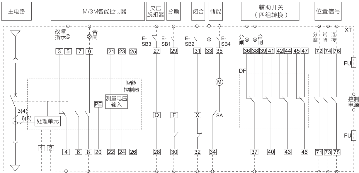
控制回路接线图 (M\3M )
