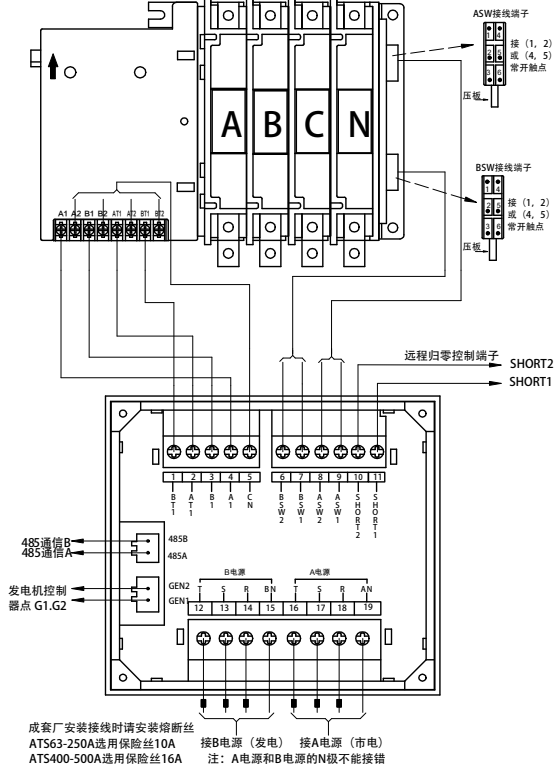
APEK2 配合 APEQ3 (500A 以下) 双电源接线示意图
