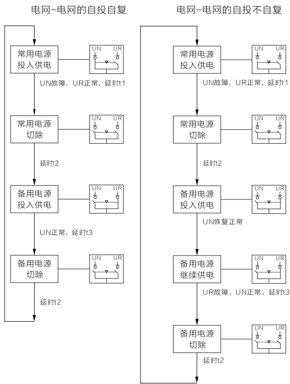
图 1 电网 – 电网自动转换逻辑
