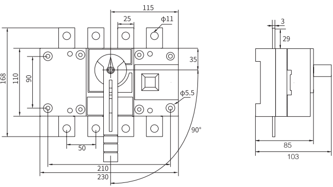
250A 4 极 外形安装尺寸图
