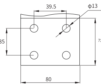
1600A 铜排辅助尺寸
