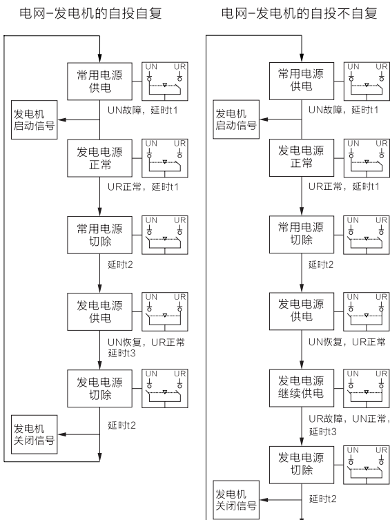
图 2 电网 – 发电自动转换逻辑
