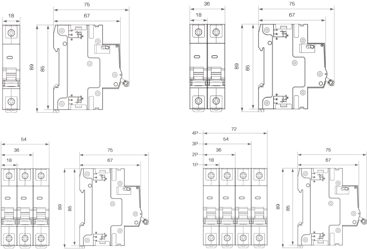
ASCB1 外观尺寸图
