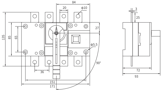
160A 4 极 外形安装尺寸图
