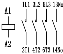
AC1-09~32/10接线图
