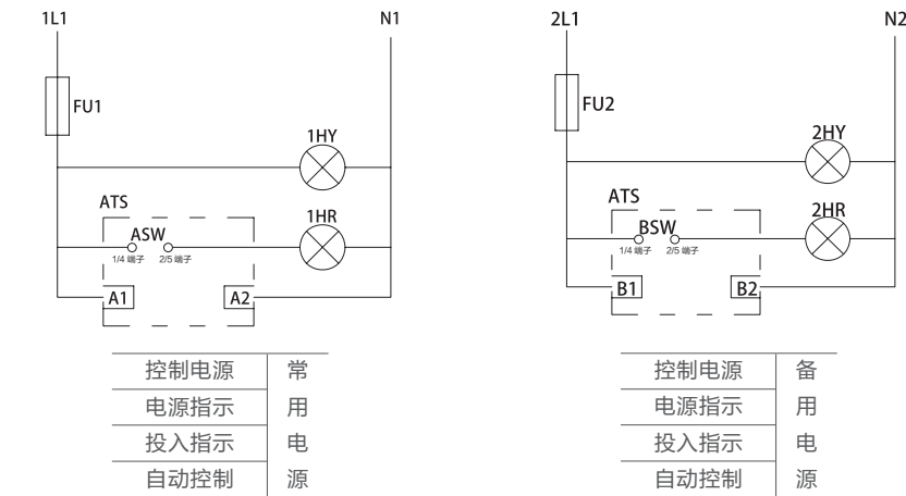
APEQ2 自投自复接线示意图
