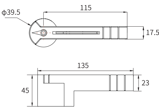
630A 及以下手柄辅助尺寸
