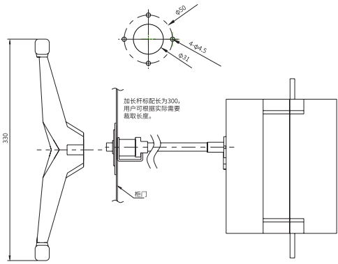
1600A-3200A 手柄辅助尺寸
