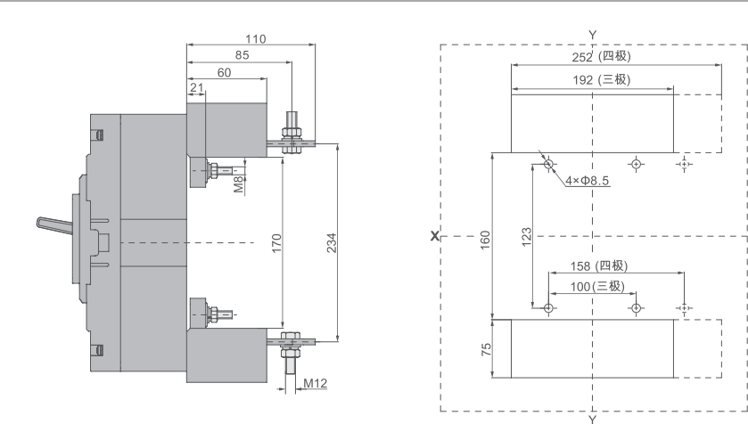
APEM6 – 630 插入式接线尺寸（三极、四极）X-X、Y-Y 三极断路器中心
