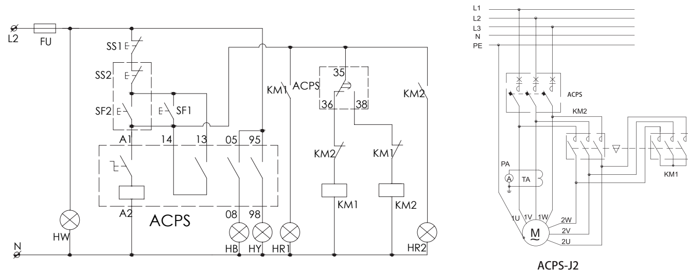
ACPS-J2 控制电路图
