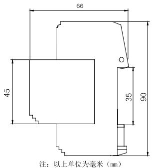
YAP1-40 外形尺寸
