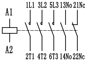
AC1-40~95/11接线图
