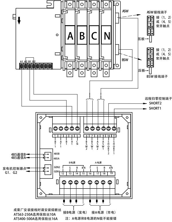
APEK2 配合 APEQ2 双电源接线示意图
