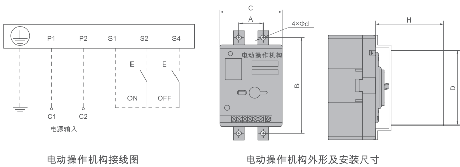
电动操作机构外形及安装尺寸图
