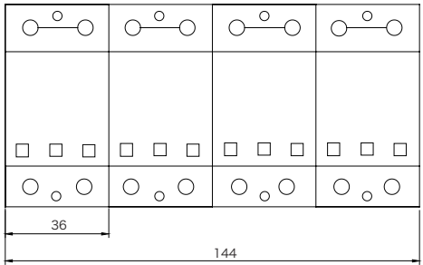
YAP1- I 25 外形尺寸
