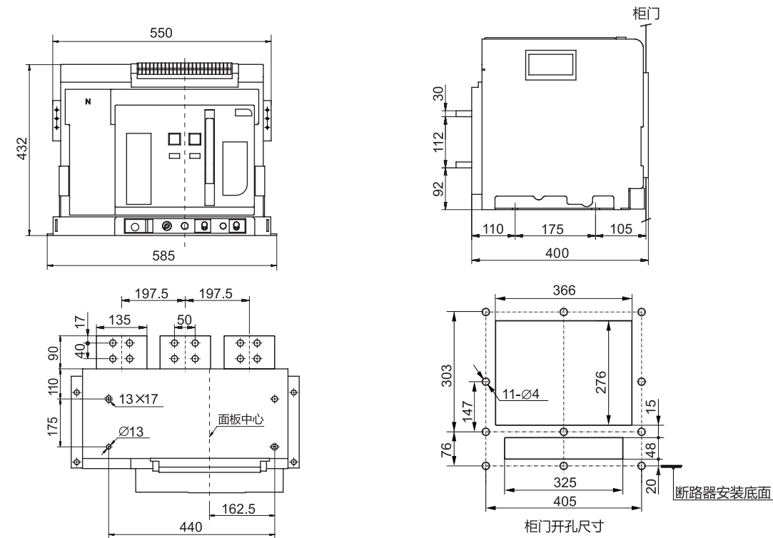
AW3-4000 抽屉式 3P
