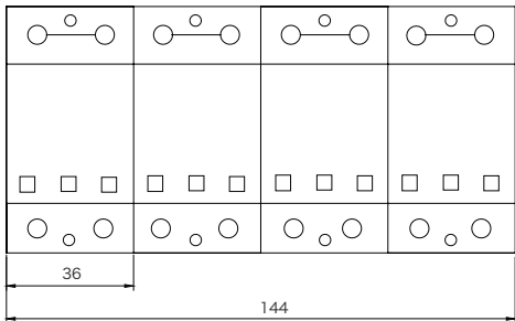
YAP1- I 15 外形尺寸
