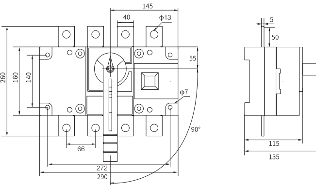
630A 4 极 外形安装尺寸图
