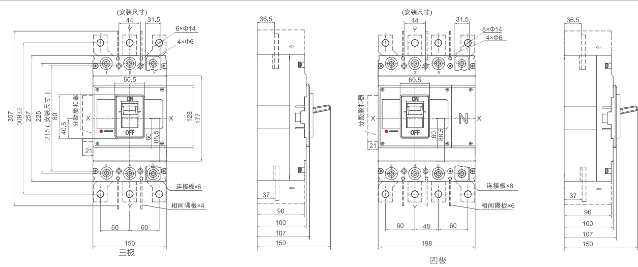
APEM6 – 400 板后接线尺寸（三极、四极）X-X、Y-Y 三极断路器中心
