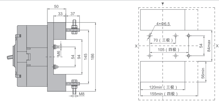
APEM6 – 400 板前接线尺寸（三极、四极）X-X、Y-Y 三极断路器中心
