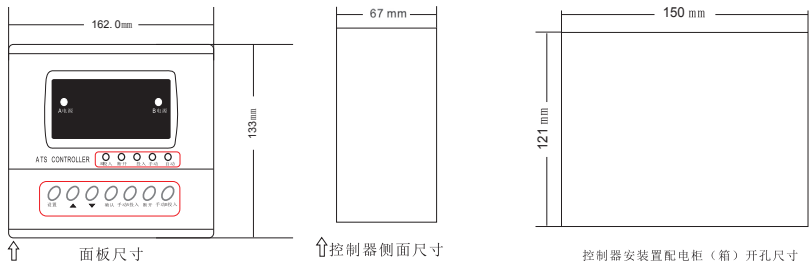
APEK2 标准控制器开孔尺寸示意图
