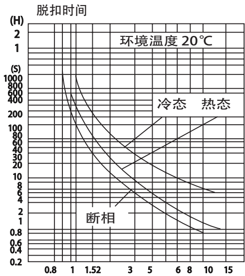
图1 整定电流倍数
