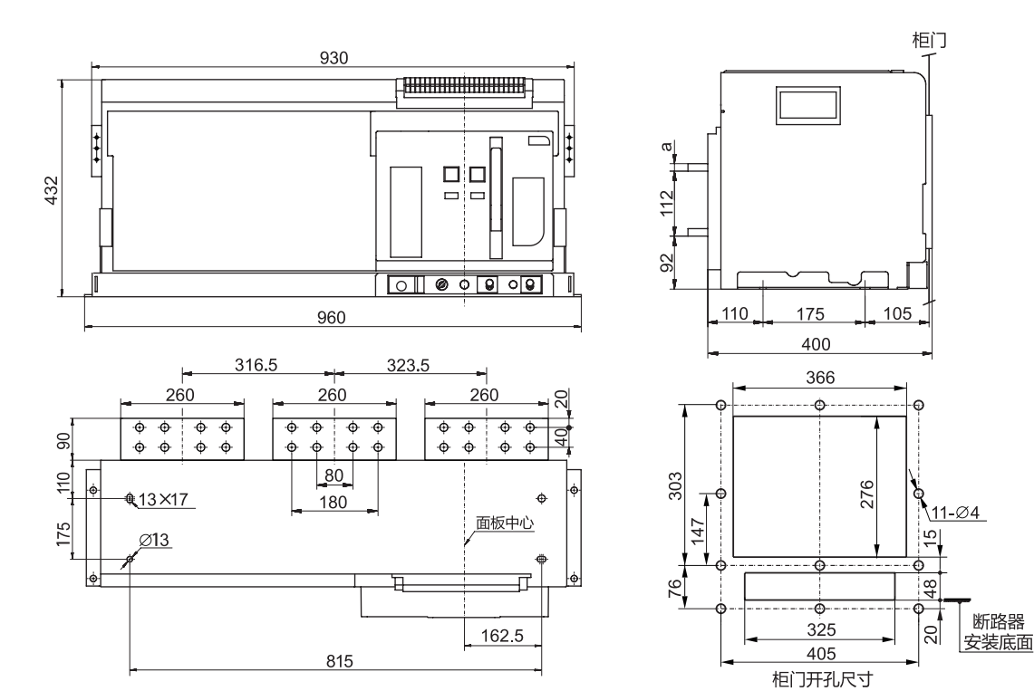
AW3-6300(6300A) 抽屉式
